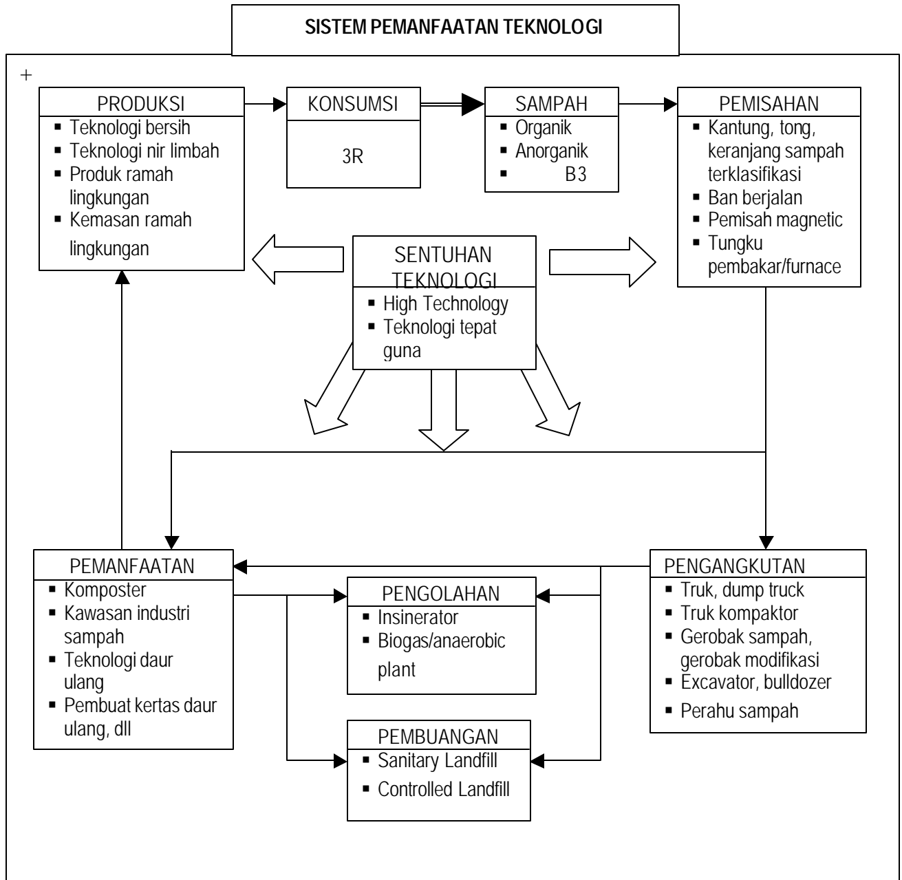
Lampiran Gambar 3. Skema Sistem
